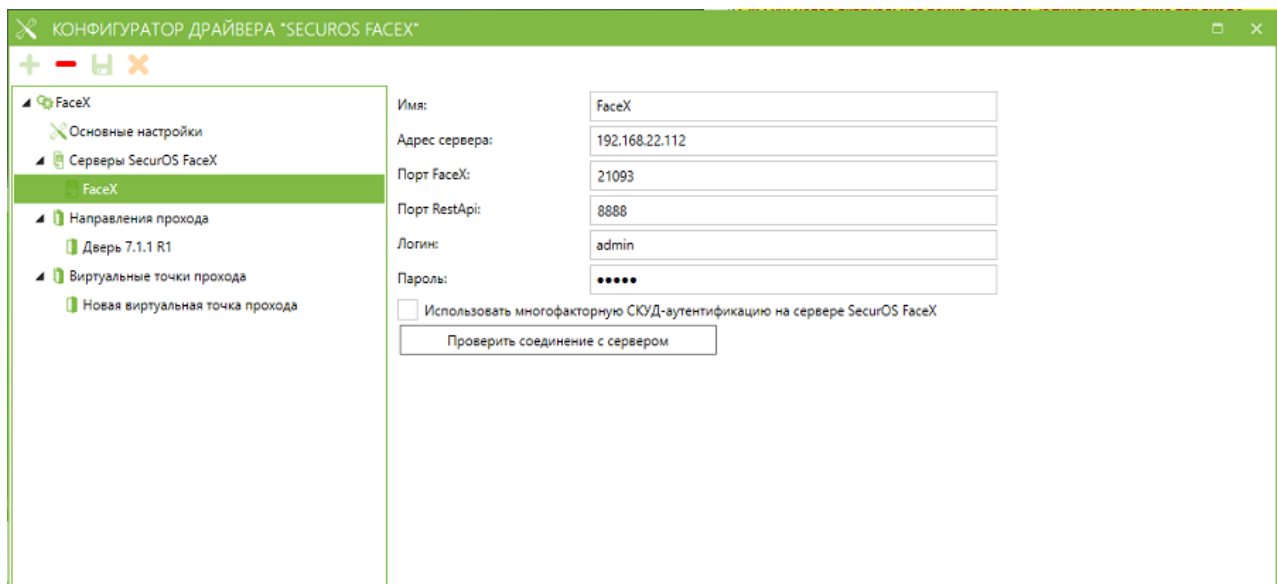
Рис. 10. Настройки подключения к серверу SecurOS FaceX
