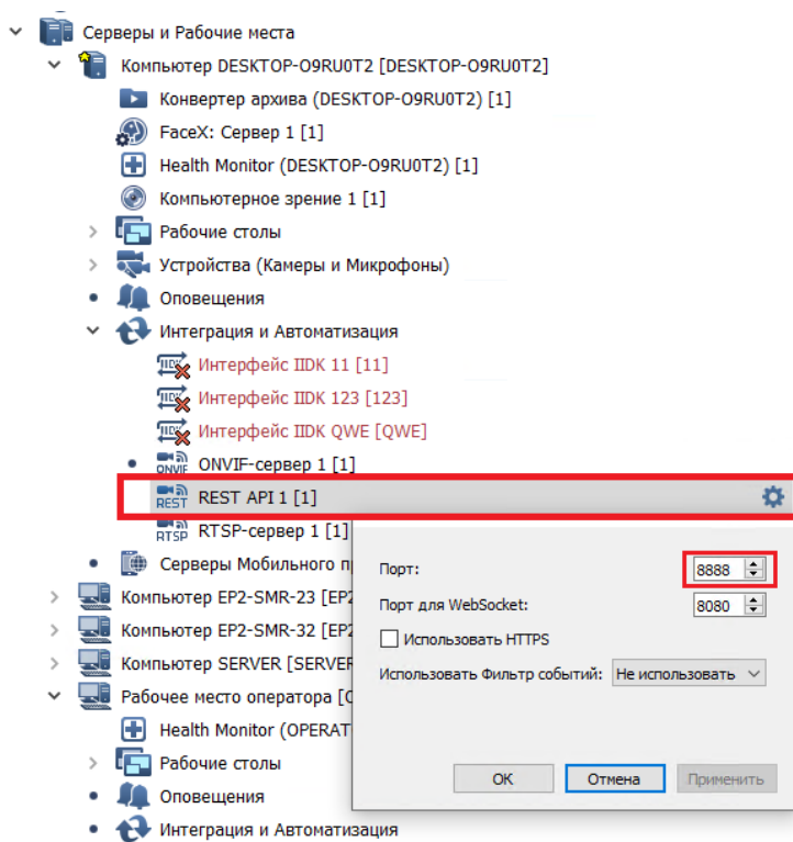
Рис. 6. Создание объекта REST API
